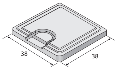
Cadre sous tampon pour grille ou plaque 30 x 30
