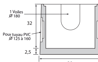
Joint caoutchouc prédécoupé pour tuyaux de Ø 80 - 100 - 110 - 125
