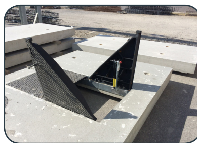
Dalle avec incorporation de tampon fonte
