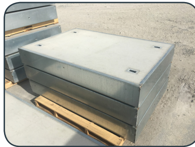
Dalle avec cadre galva
